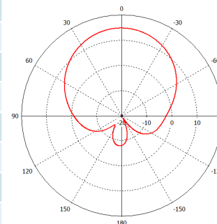
790-960MHz
