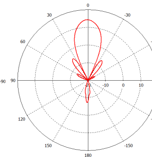
1710-2170MHz
