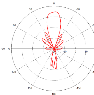
2490-2690MHz
